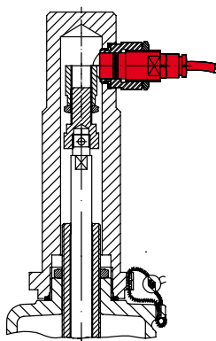
Detector inductivo
