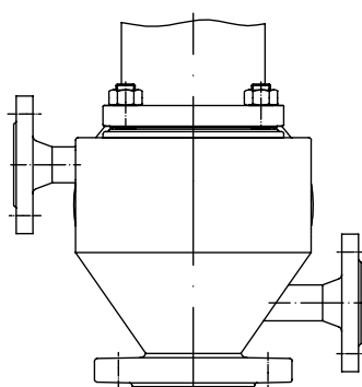
Cámara calefacción
