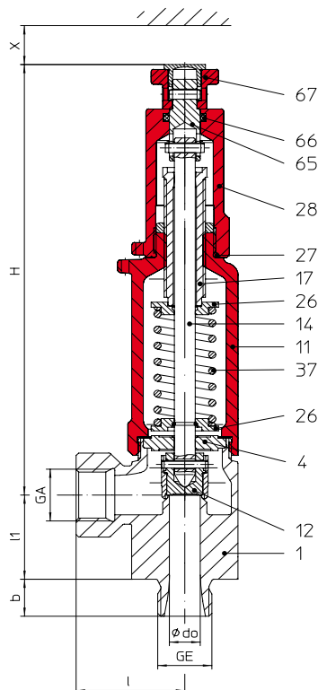
Fig. ... 961 capuchón cerrado
