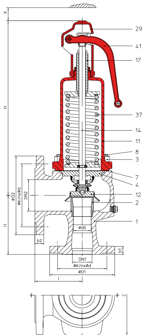
Fig. ... 904 capuchón abierto con palanca, bonete cerrado
