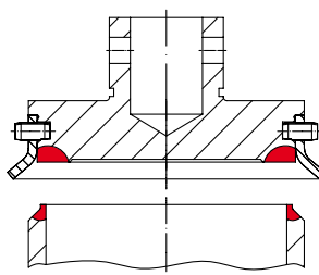
Asiento 1.4571 / Stellite No. 21 Disco 1.4571 / Stellite No. 6 Asiento SA479Gr.316Ti / Stellite No. 21 (SAFE-SN ANSI) Disco SA479Gr.316Ti / Stellite No. 6 (SAFE-SN ANSI) y ayuda levantamiento desmontable
