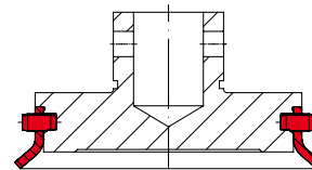
Disco de ruptura (Dimensión ver página 46)
