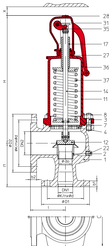
Fig. ... 901 capuchón cerrado con palanca, bonete cerrado
